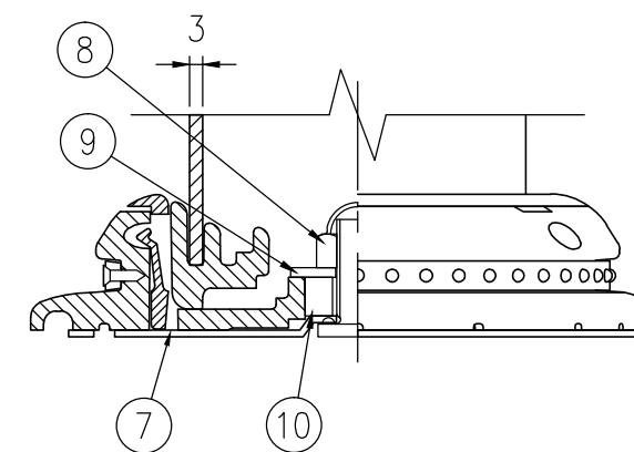
A-A半断面図 S=1/2
