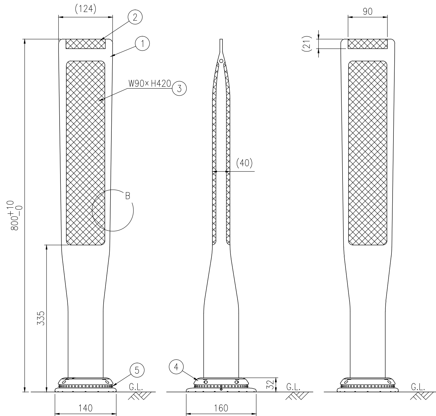
設置図 S=1/5
