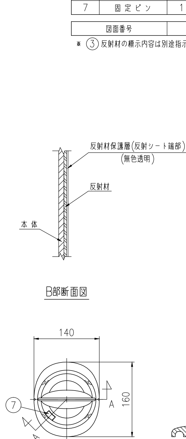
平面図 S=1/5
