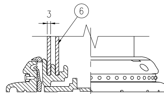
A-A半断面図 S=1/2
