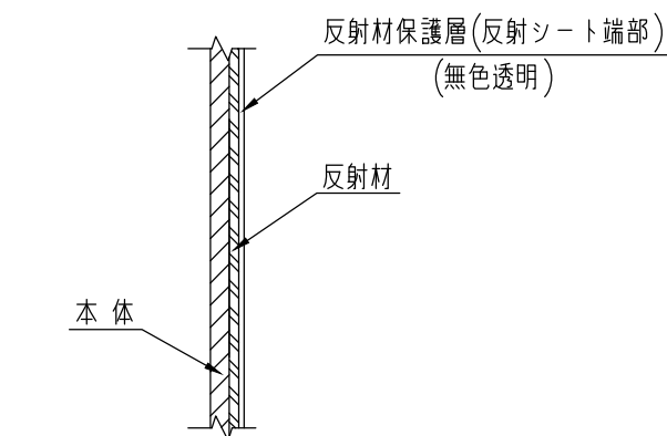
B部断面図
