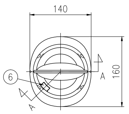
平面図 S=1/5
