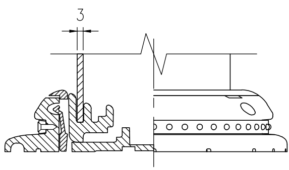
A-A半断面図 S=1/2
