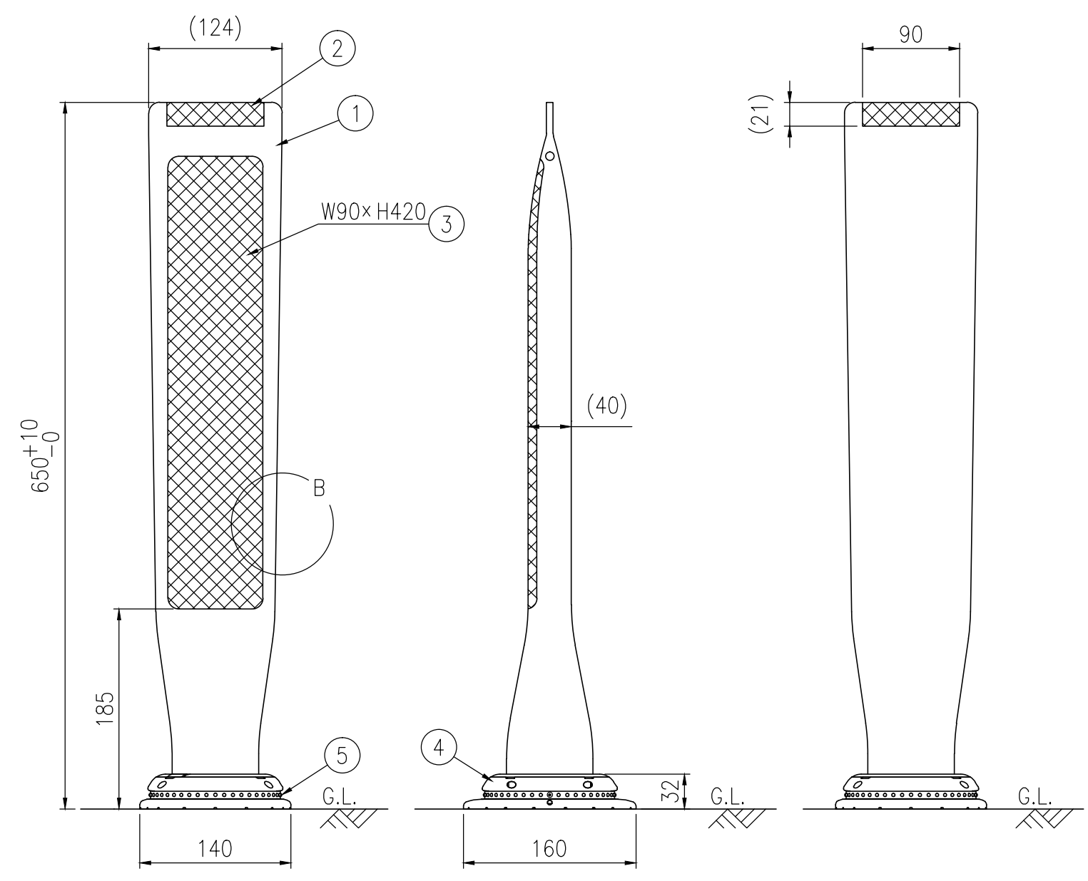
設置図 S=1/5
