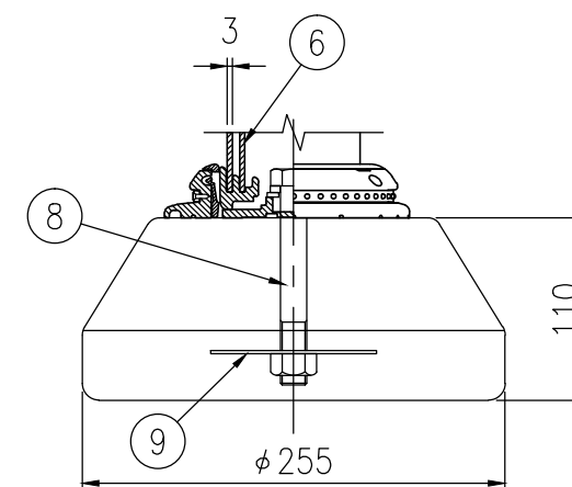
A-A半断面図 S=1/5
