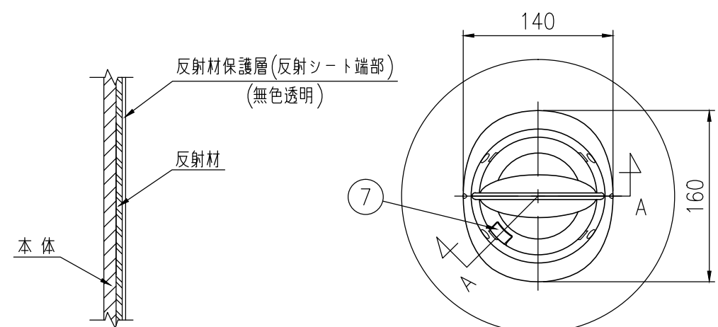
平面図 S=1/5
