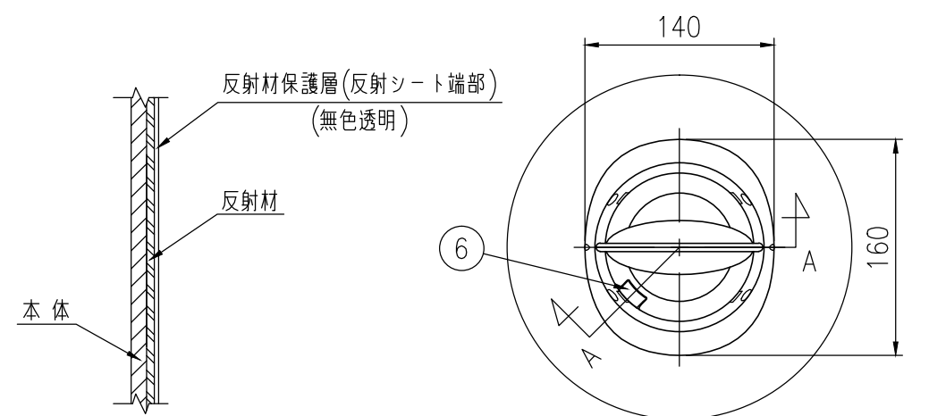
B部断面図
