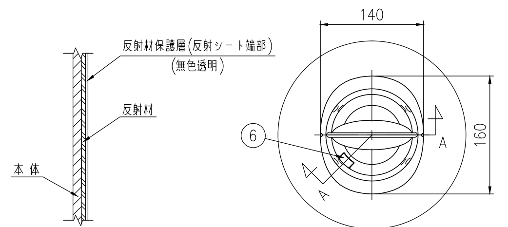
平面図 S=1/5
