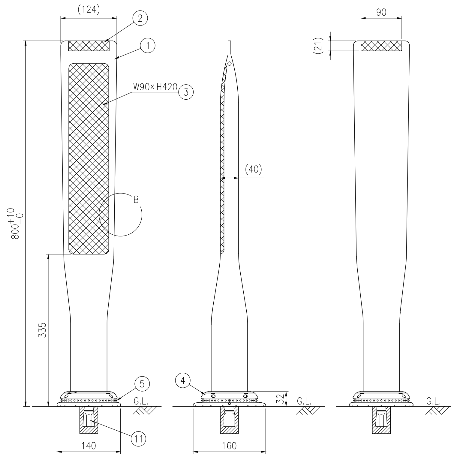
設置図 S=1/5
