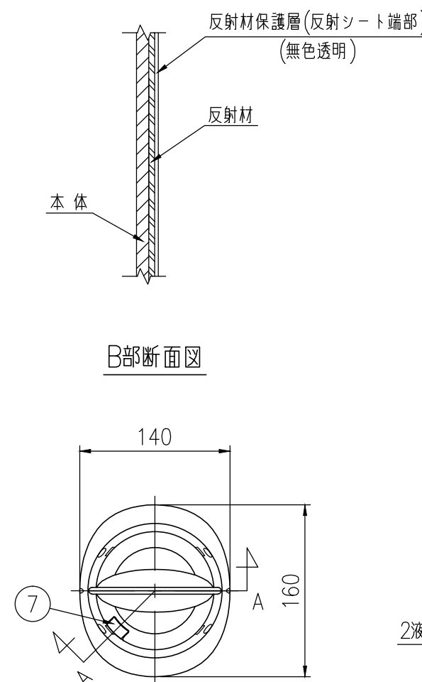
平面図 S=1/5
