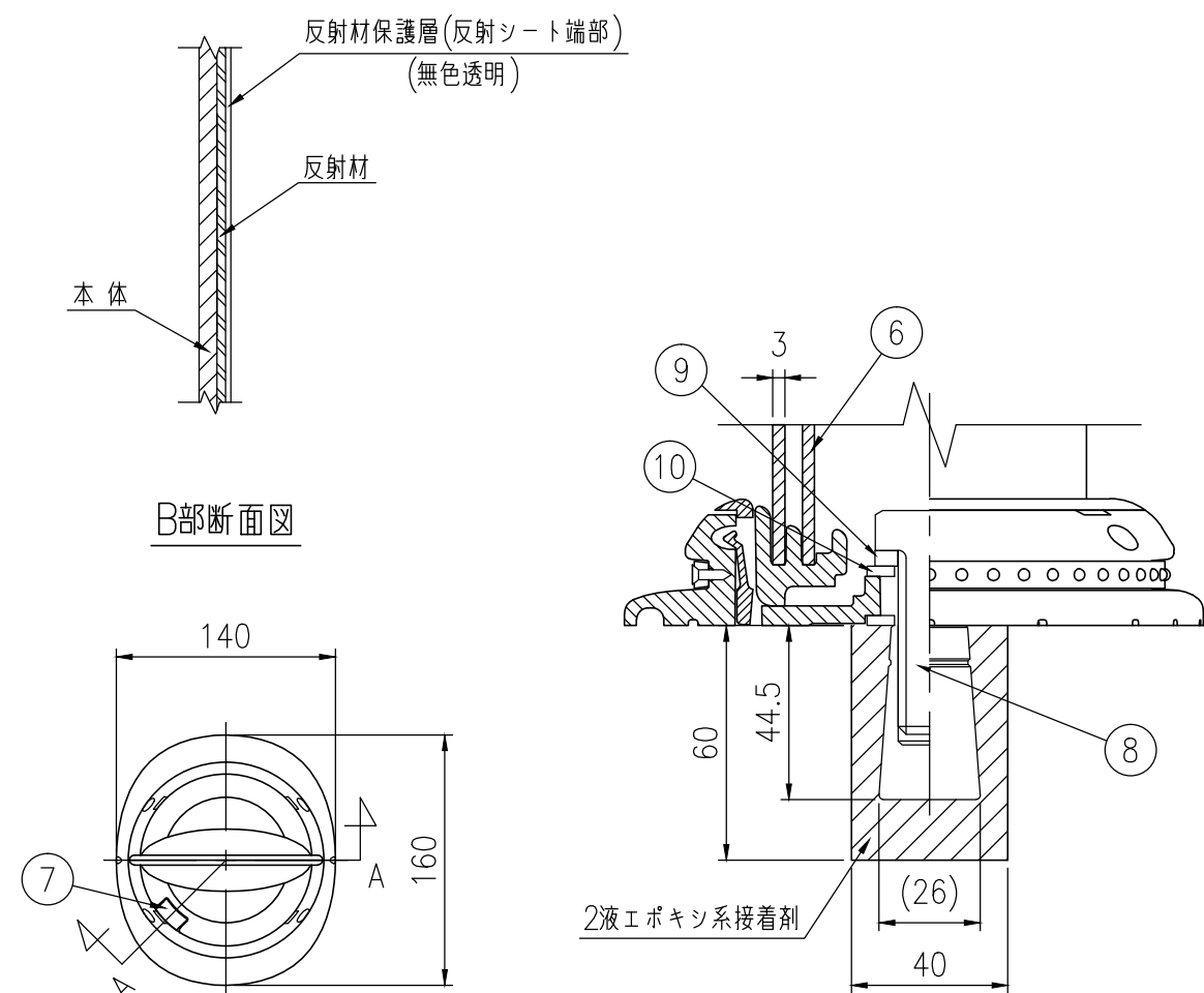
平面図 S=1/5
