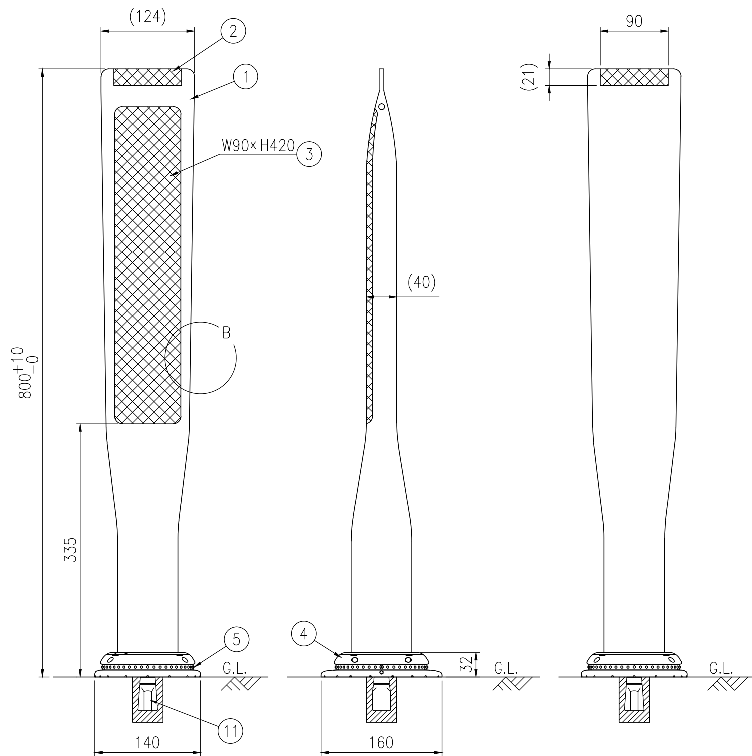
設置図 S=1/5
