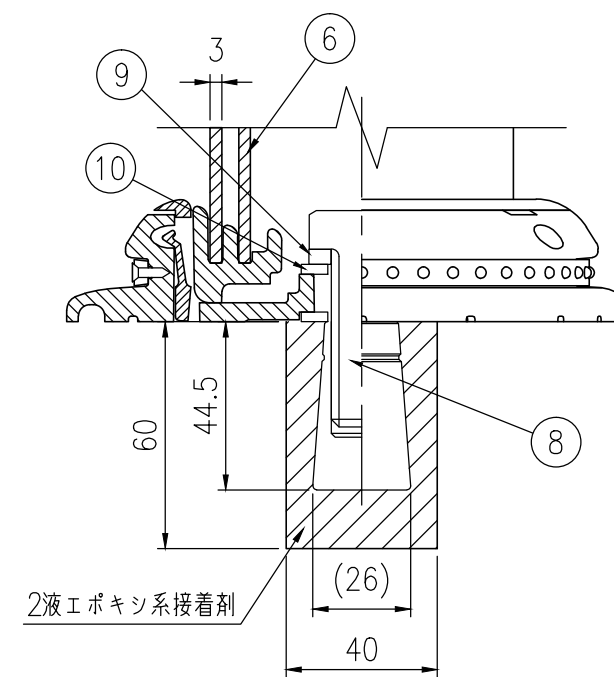
A-A半断面図 S=1/2
