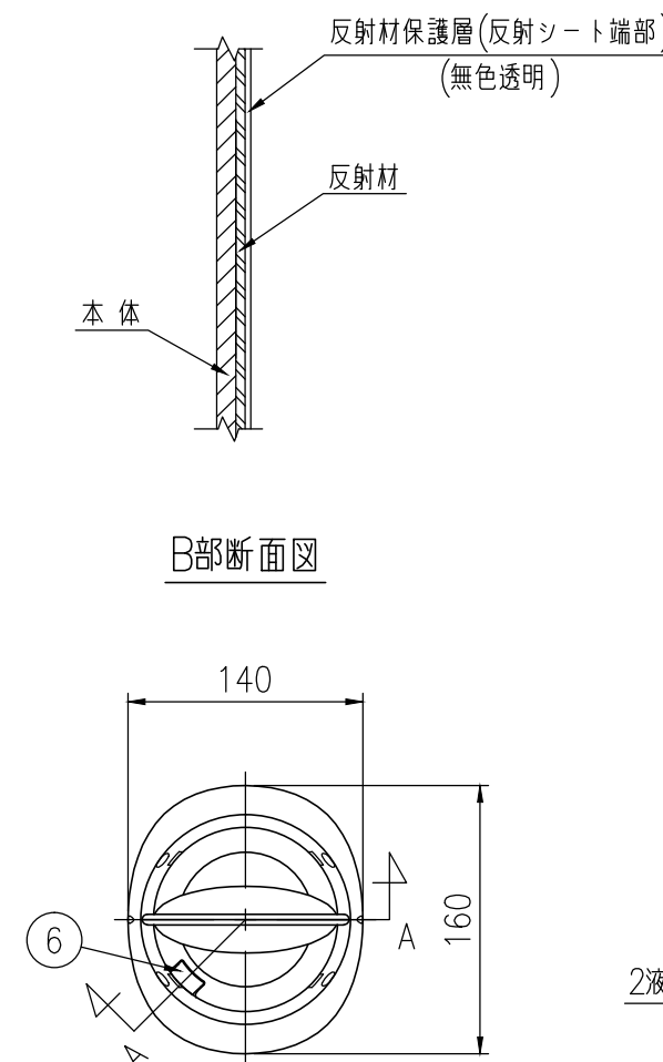
平面図 S=1/5
