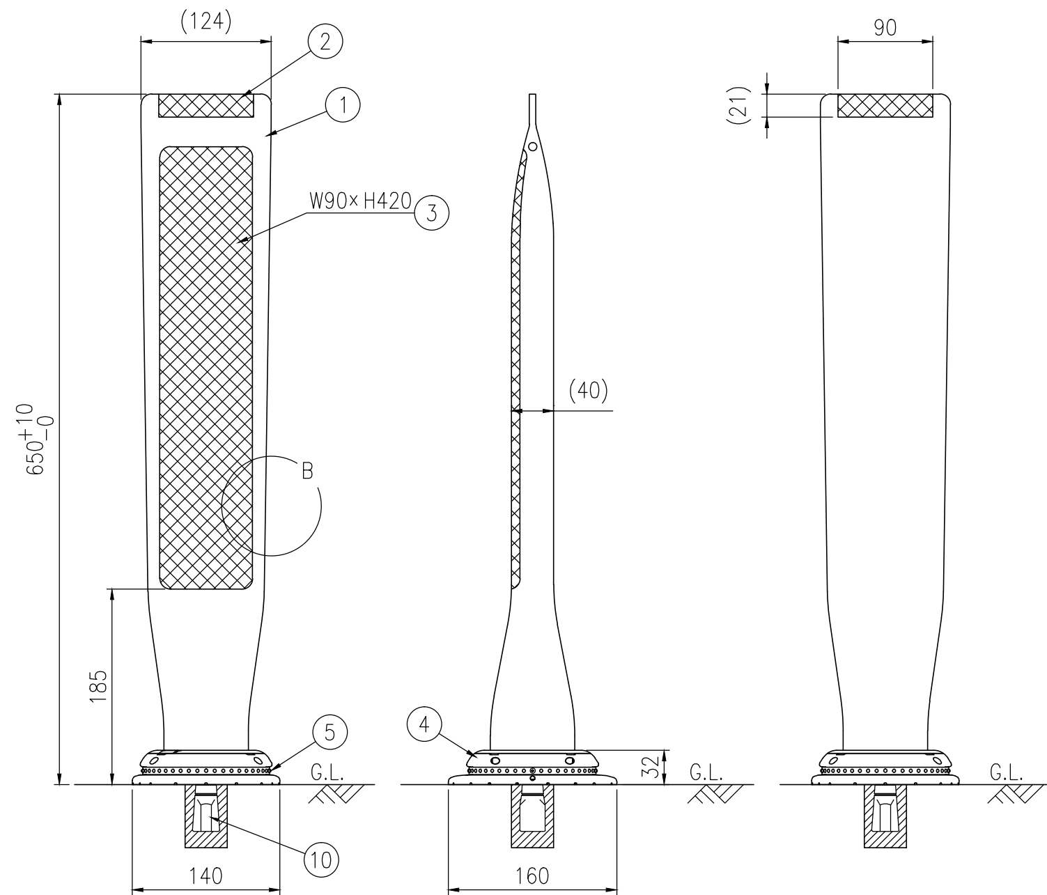
設置図 S=1/5
