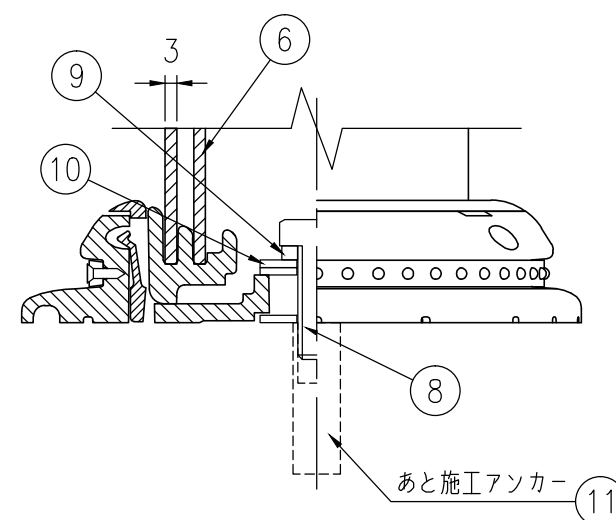
A-A半断面図 S=1/2
