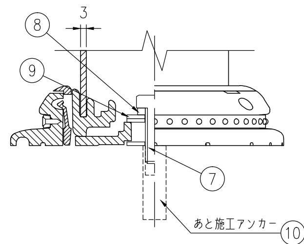
A-A半断面図 S=1/2
