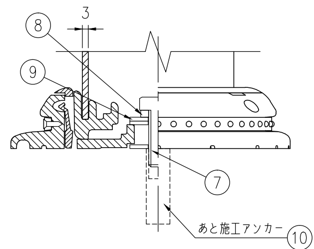
A-A半断面図 S=1/2
