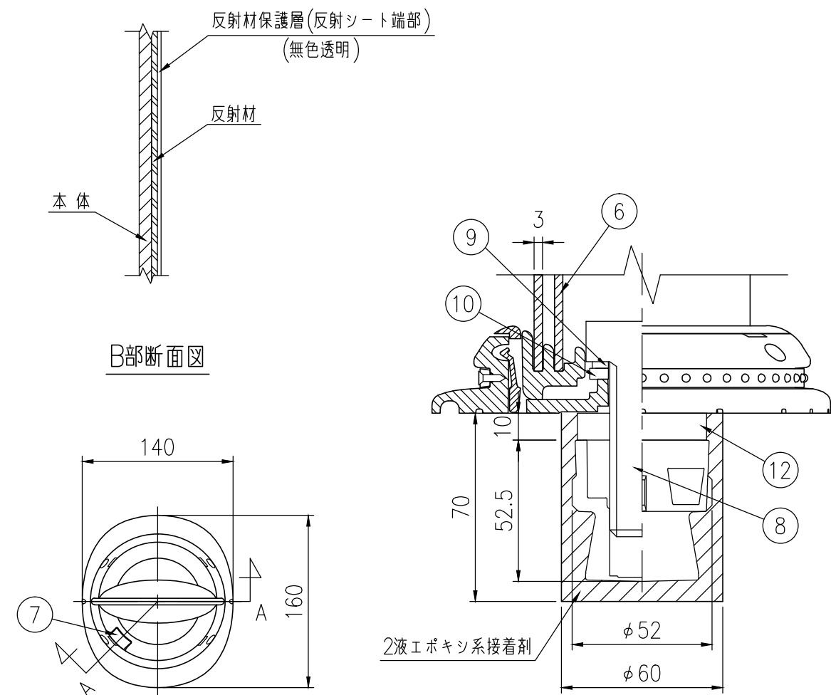
平面図 S=1/5
