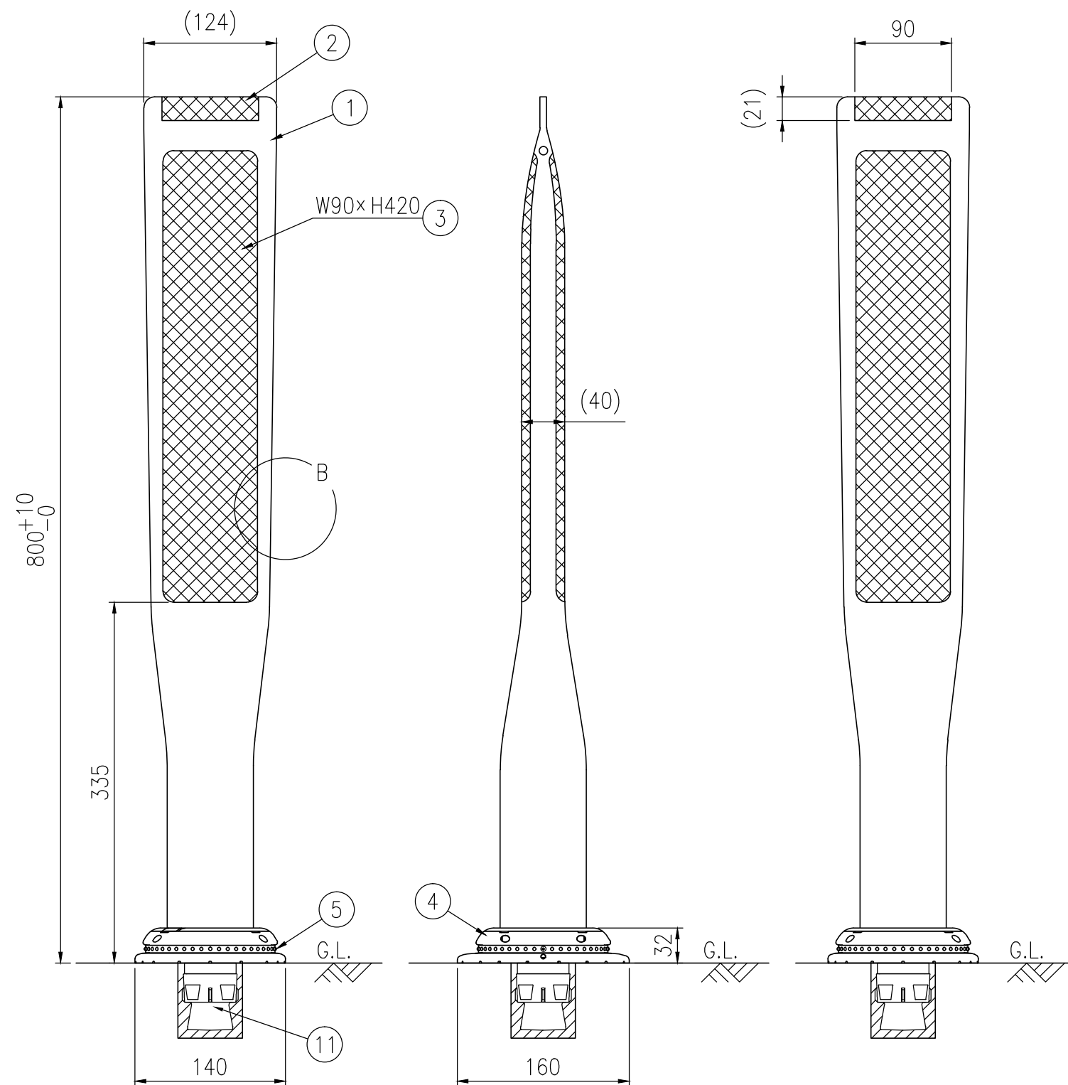
設置図 S=1/5
