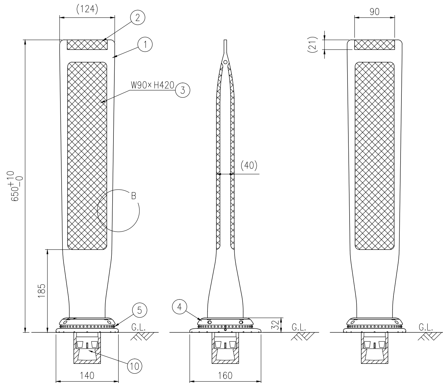
設置図 S=1/5
