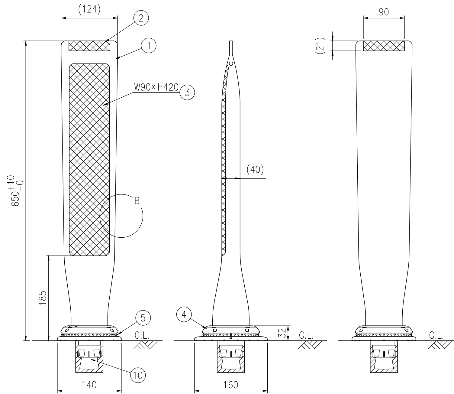
設置図 S=1/5
