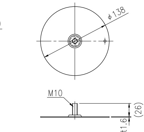
8部スチールスペーサー詳細図 S=1/4
