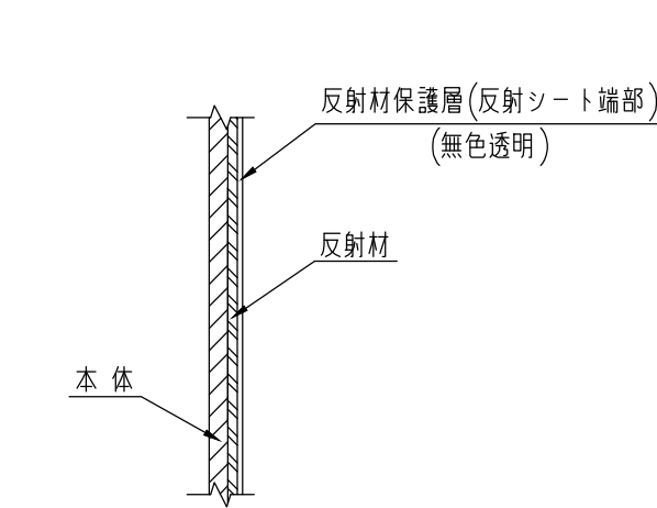
B部断面図
