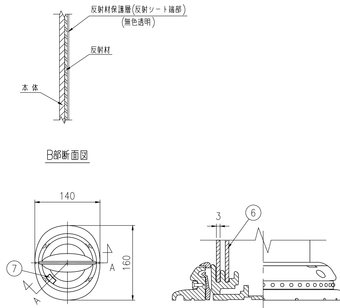
平面図 S=1/5
