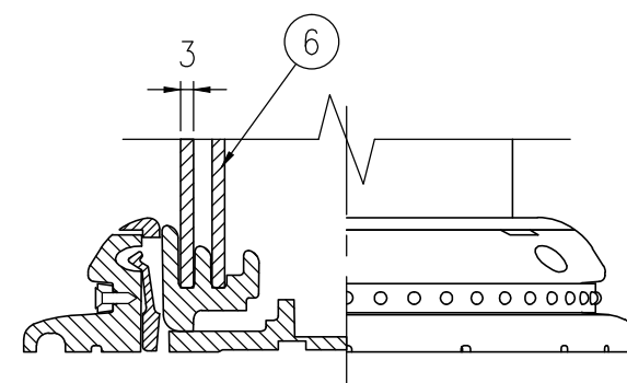
A-A半断面図 S=1/2
