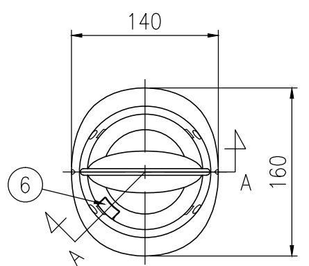
平面図 S=1/5
