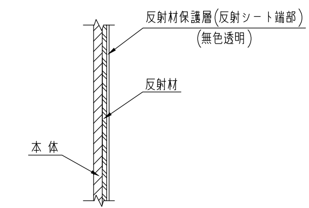
B部断面図
