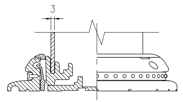
A-A半断面図 S=1/2
