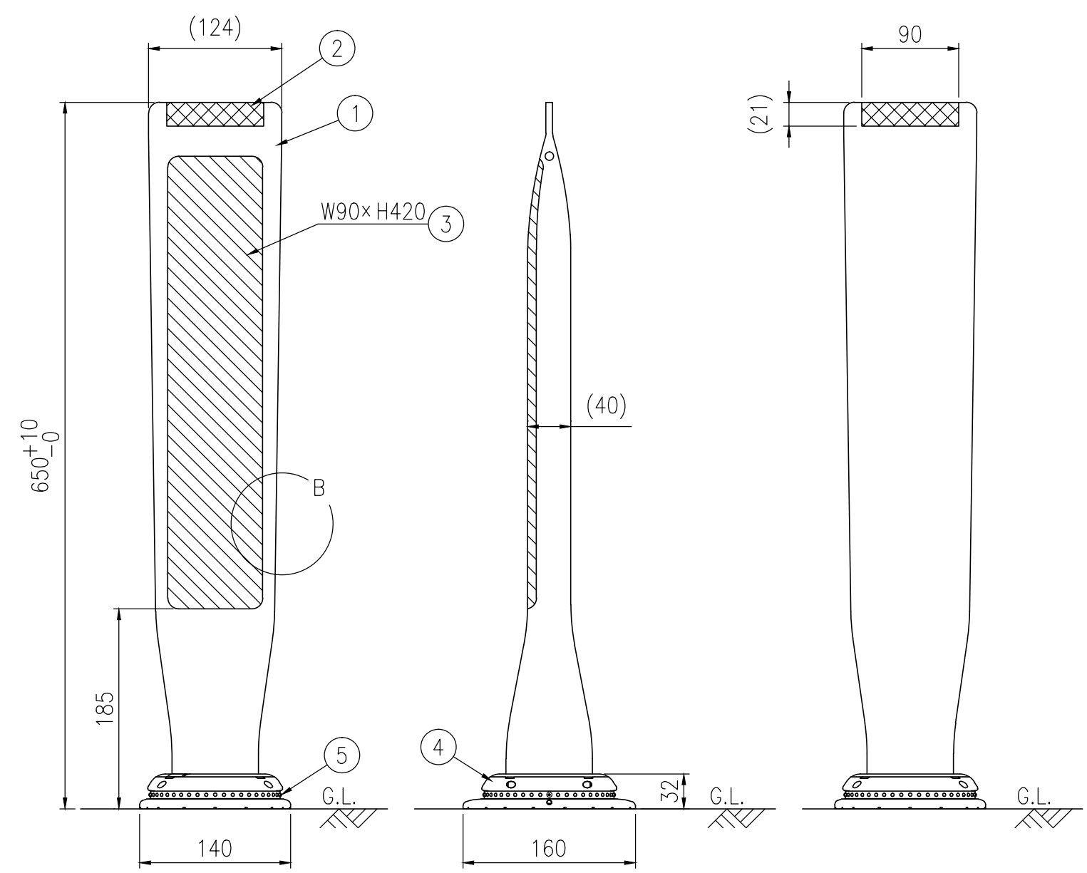
設置図 S=1/5
