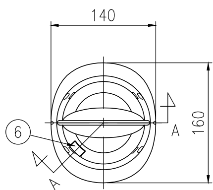
平面図 S=1/5
