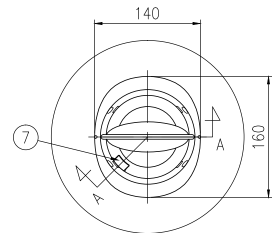
平面図 S=1/5
