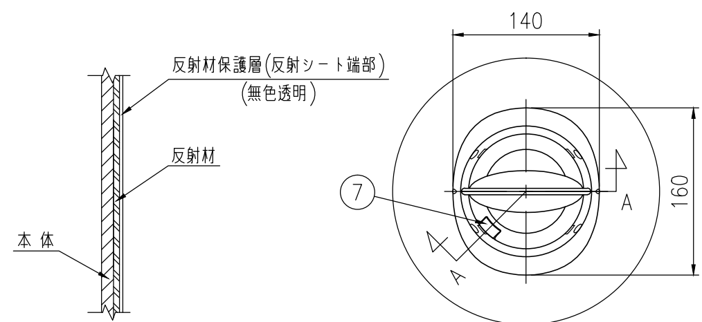
B部断面図
