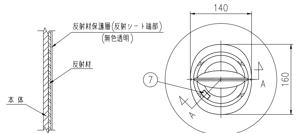
平面図 S=1/5
