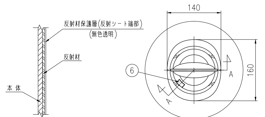
平面図 S=1/5
