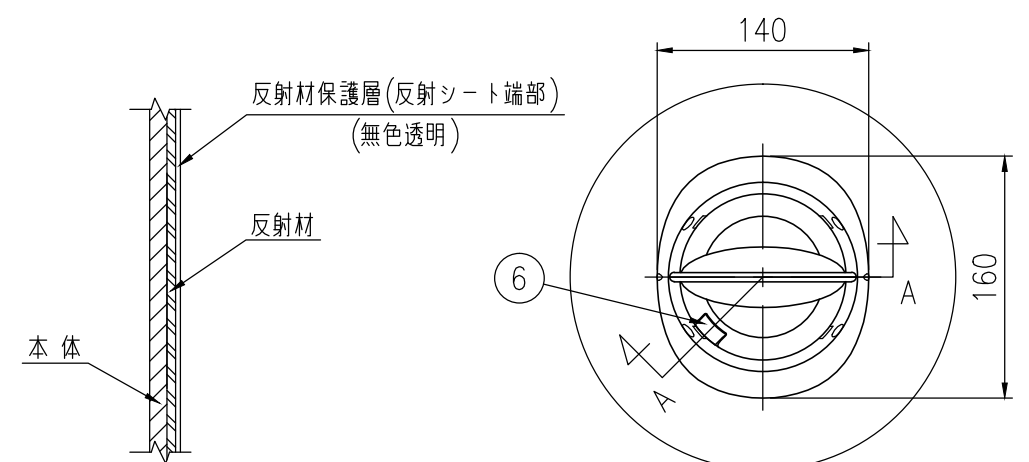
平面図 S=1/5
