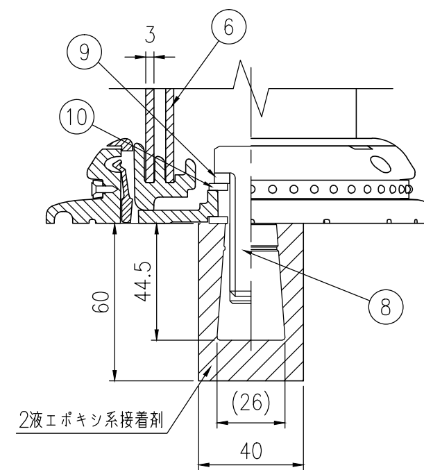
A-A半断面図 S=1/2
