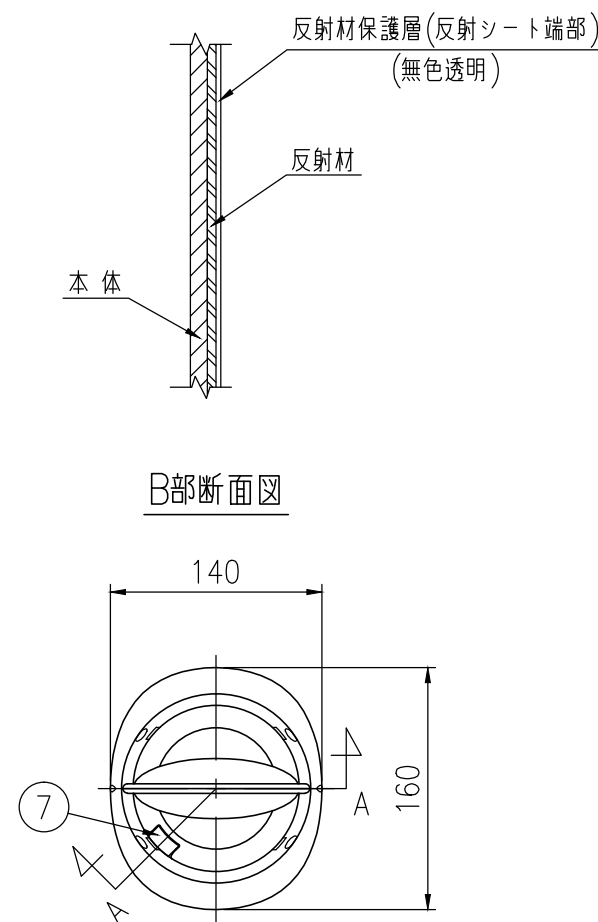
平面図 S=1/5
