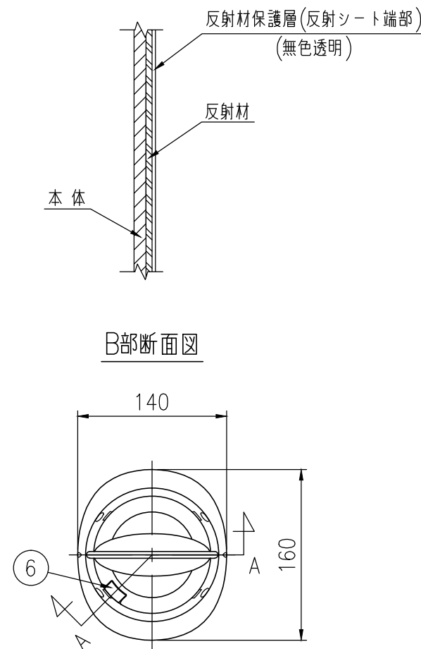
平面図 S=1/5
