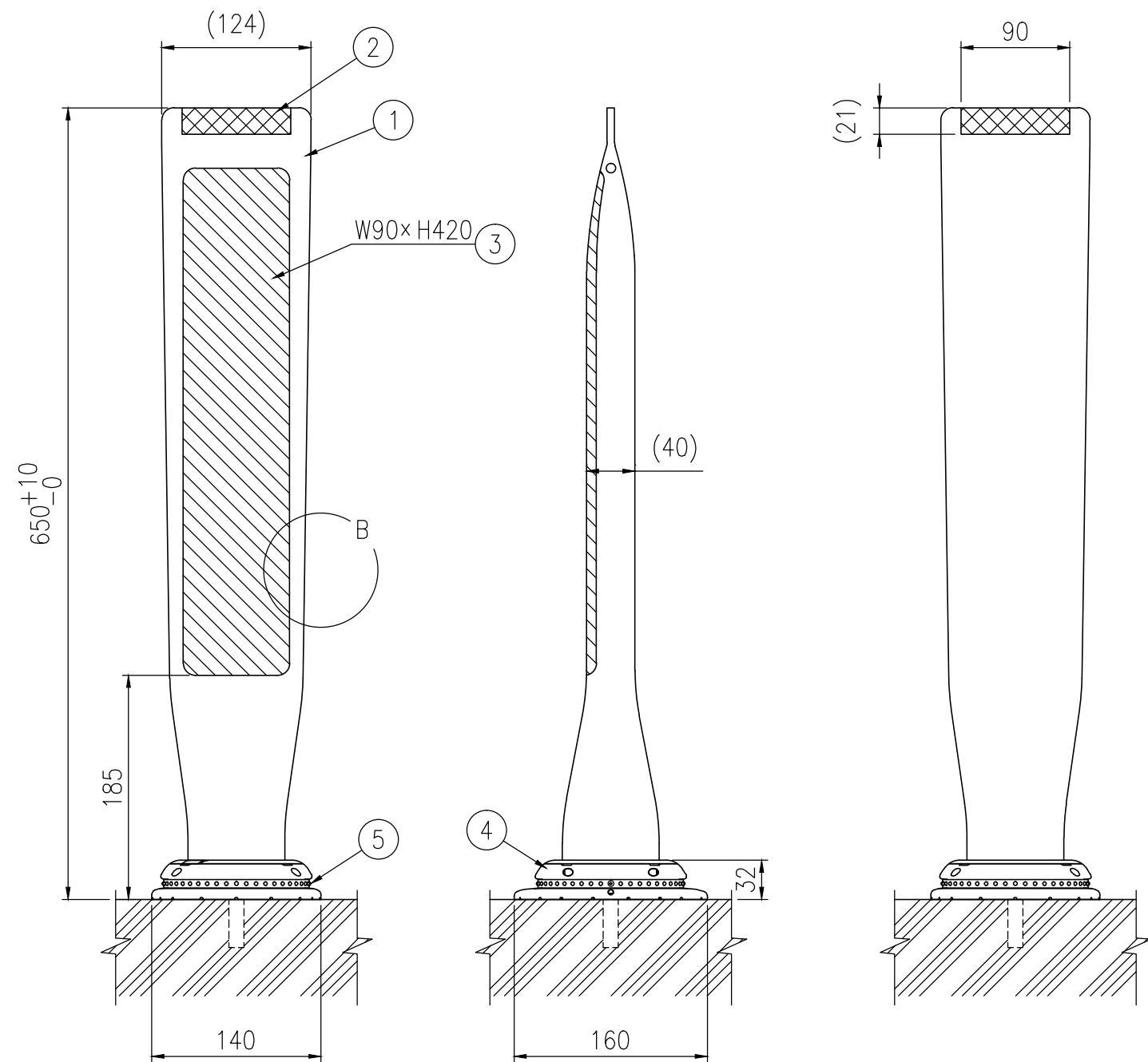
設置図 S=1/5
