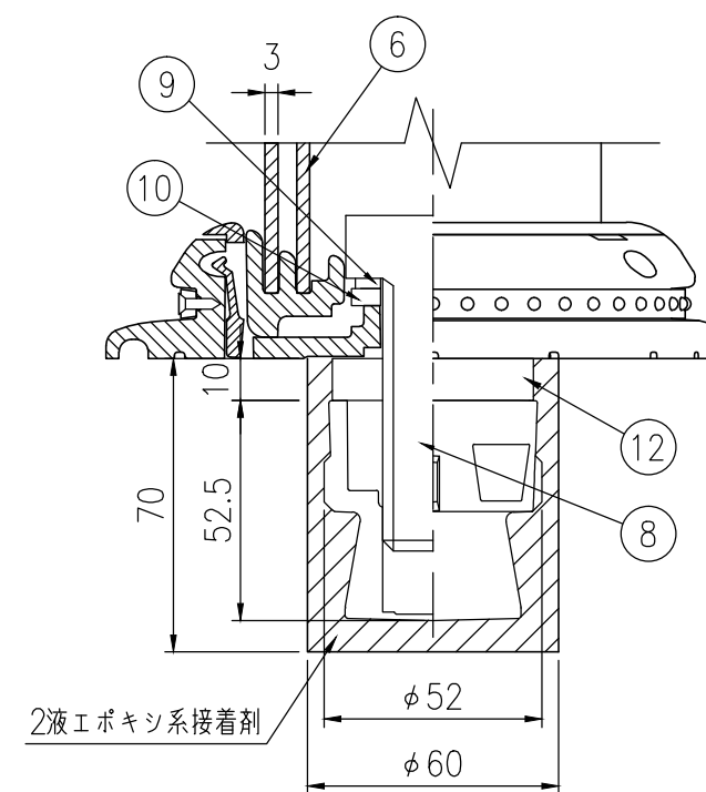
A-A半断面図 S=1/2
