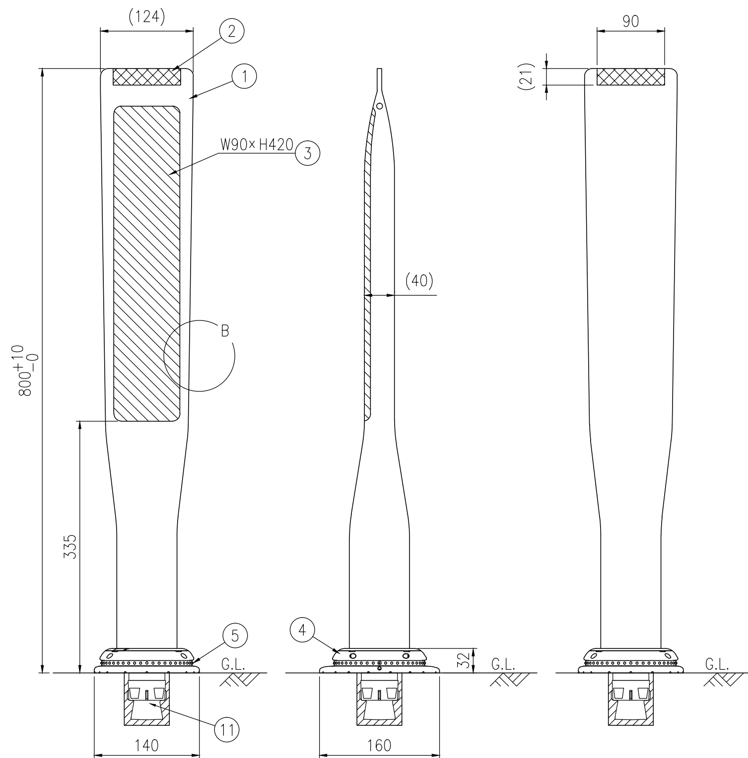
設置図 S=1/5
