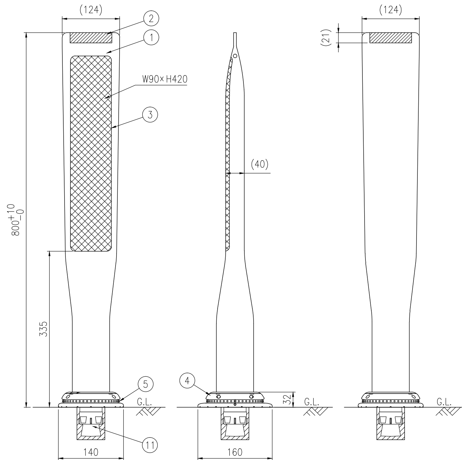
設置図 S=1/5
