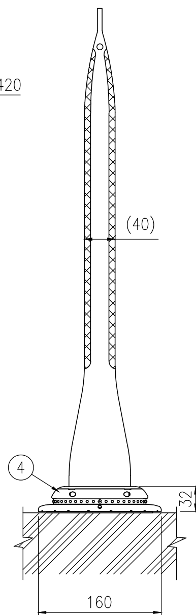
設置図 S=1/5
