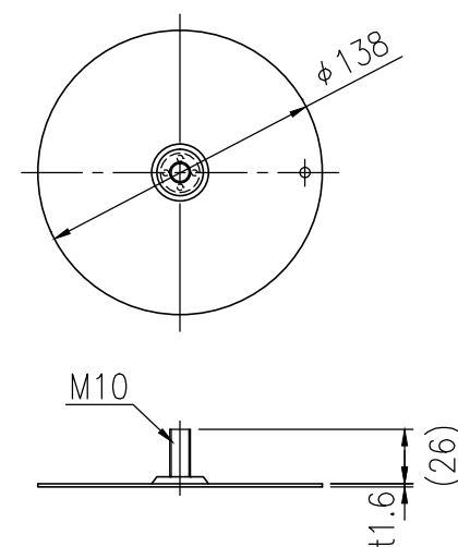
⑦ スチールスペーサー詳細図 S=1/4
