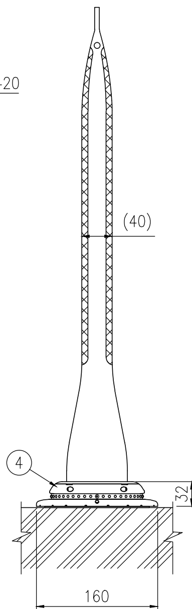
設置図 S=1/5
