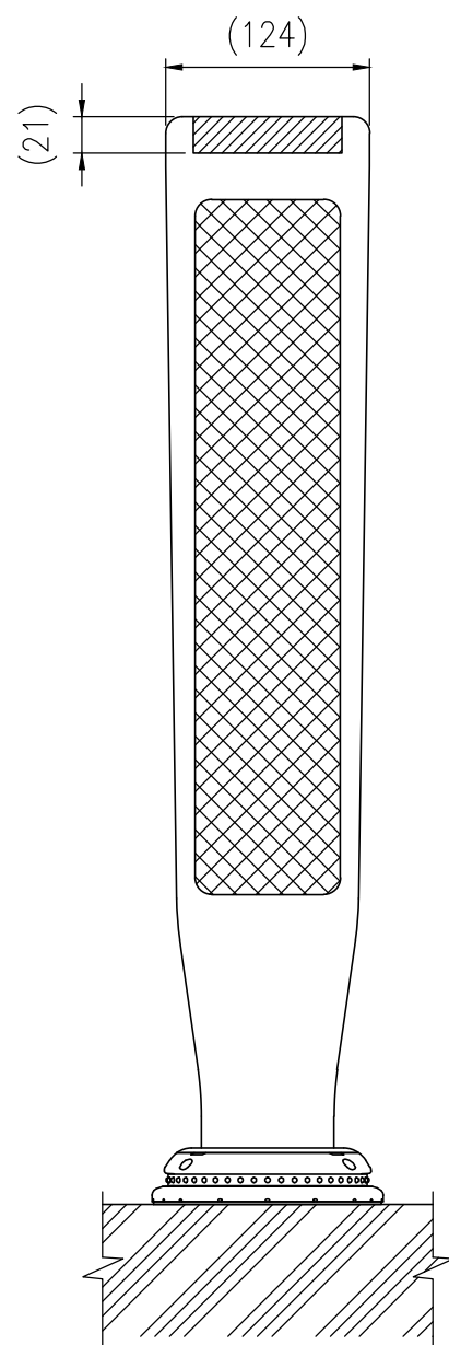
⑦ スチールスペーサー詳細図 S=1/4
