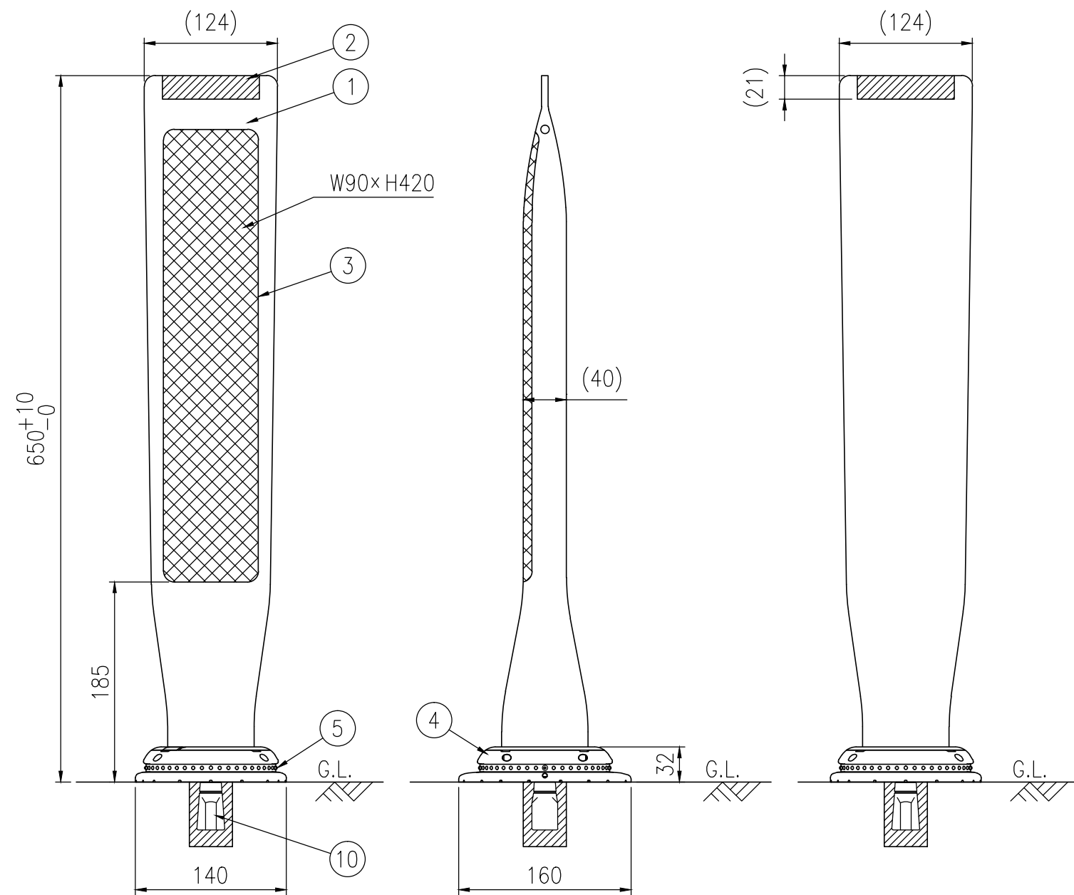
設置図 S=1/5
