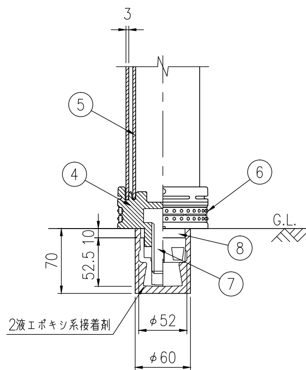
ベース部詳細図 S=1/4
