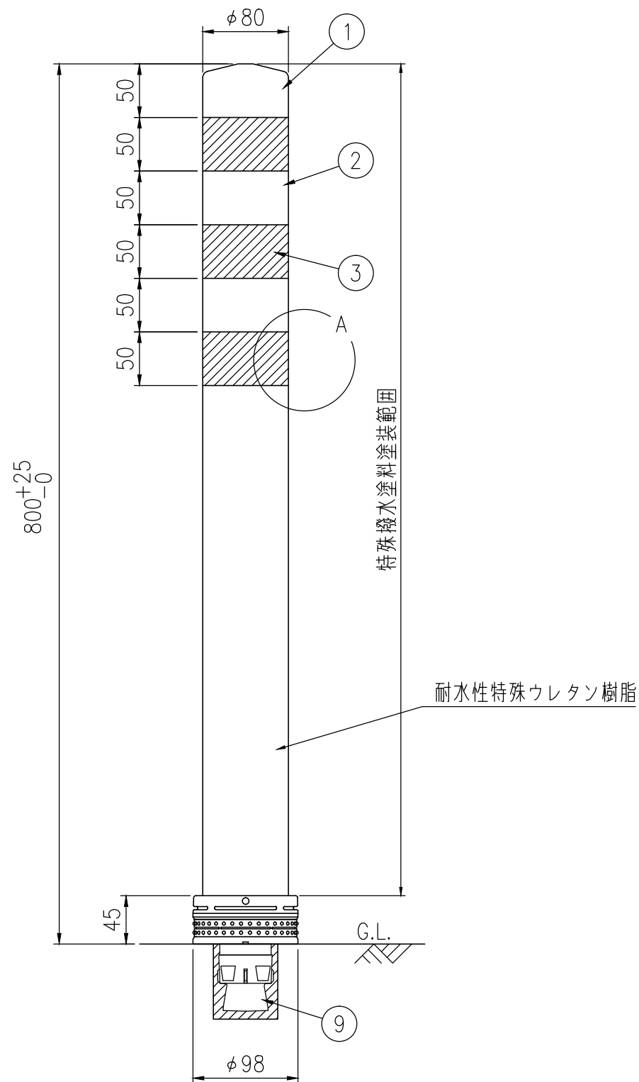
設置図 S=1/5
