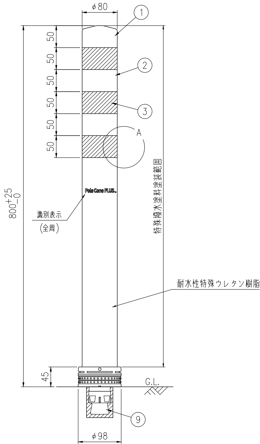
設置図 S=1/5
