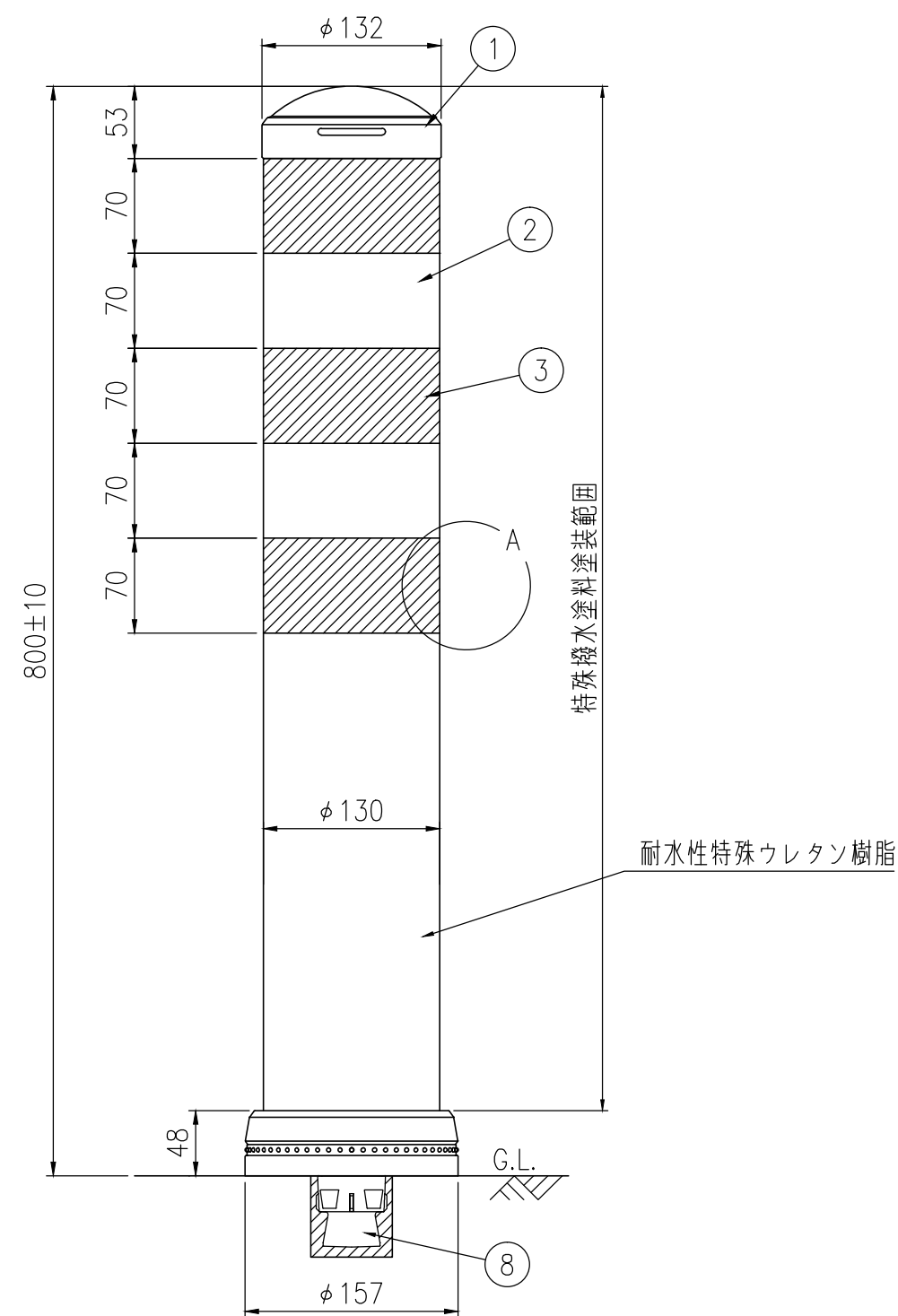
設置図 S=1/5
