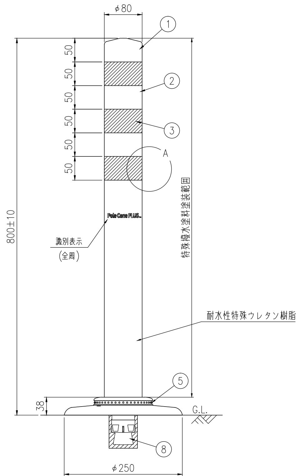
設置図 S=1/5
