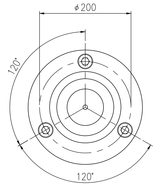
上面図 S=1/5
