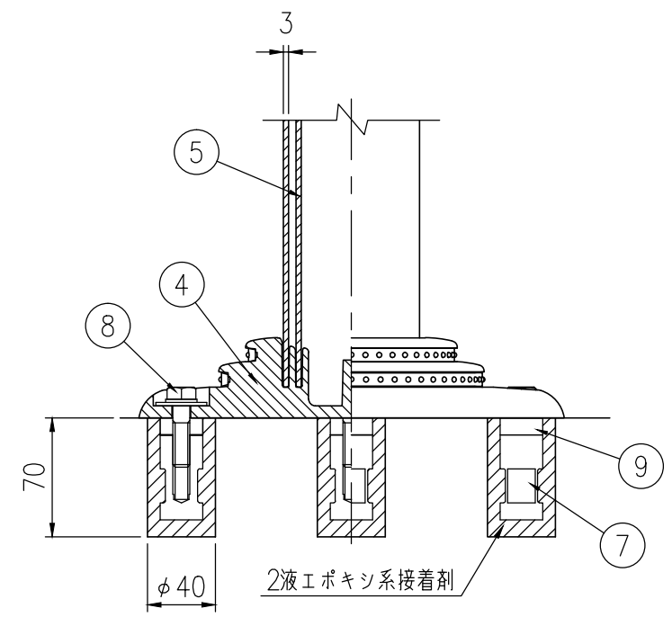
ベース部詳細図 S=1/4
