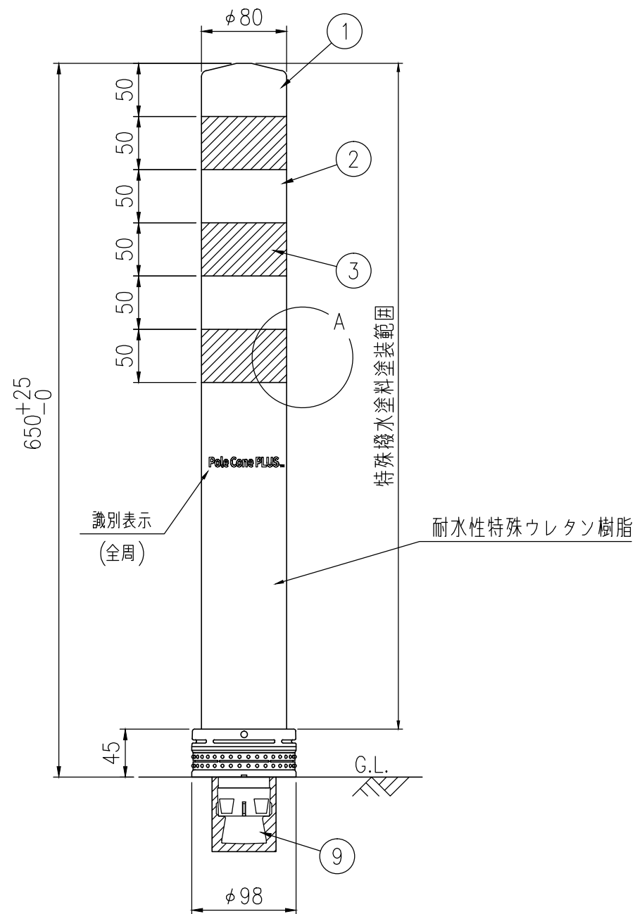
設置図 S=1/5
