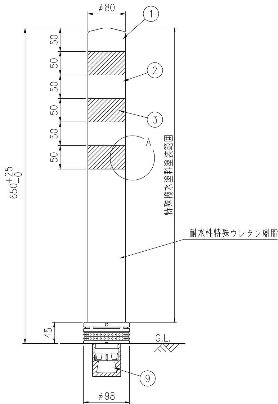
設置図 S=1/5
