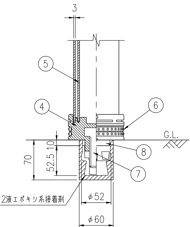
ベース部詳細図 S=1/4
