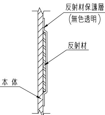
A部断面図
