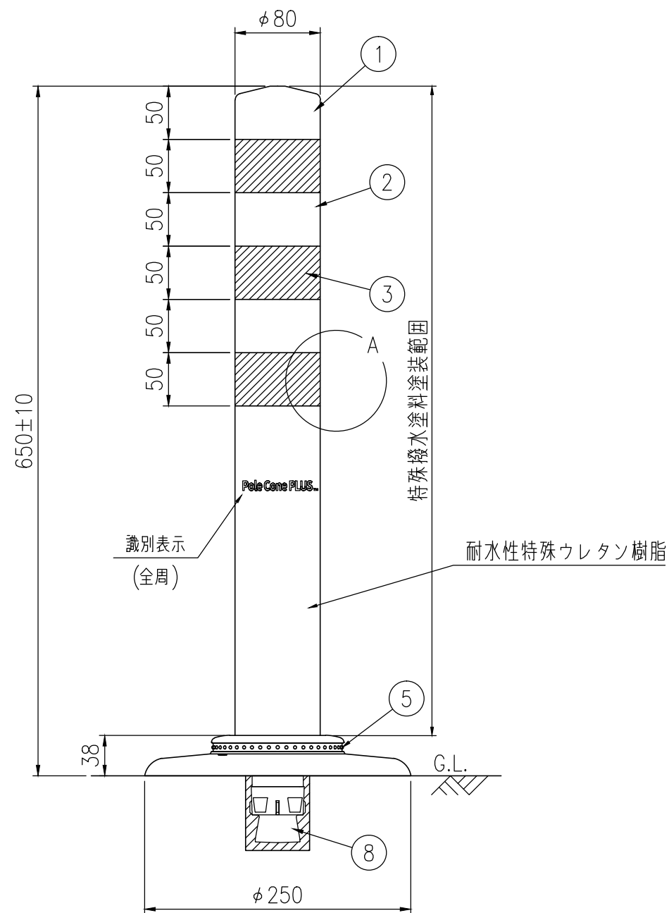
設置図 S=1/5
